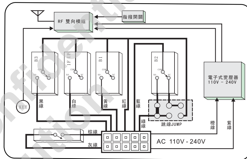
地下3樓方塊圖
