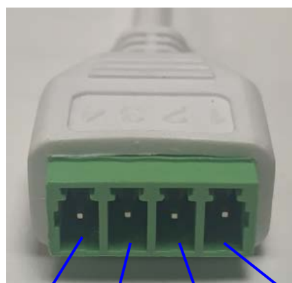
端子定義 ( 由左至右 ):
